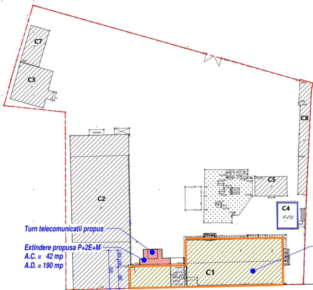
Figura 3 Schița amplasamentului – Terenul și clădirile existente.
